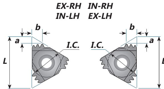
Mehrzahn | Multi-tooth
